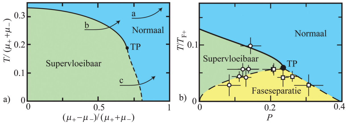
Figuur 4 Fasediagram voor een homogeen Fermi-mengsel met resonante interacties, bepaald met a) BCS-theorie, en met b) renormalisatietechnieken [3]. De continue faseovergang wordt weergegeven met een doorgetrokken lijn, de discontinue overgang met een onderbroken lijn. In b) is alleen de doorgetrokken lijn berekend, de stippellijnen zijn geschetst. De Fermi-temperatuur T_{F\sigma} is per definitie evenredig met N_{\sigma}^{2/3} .
